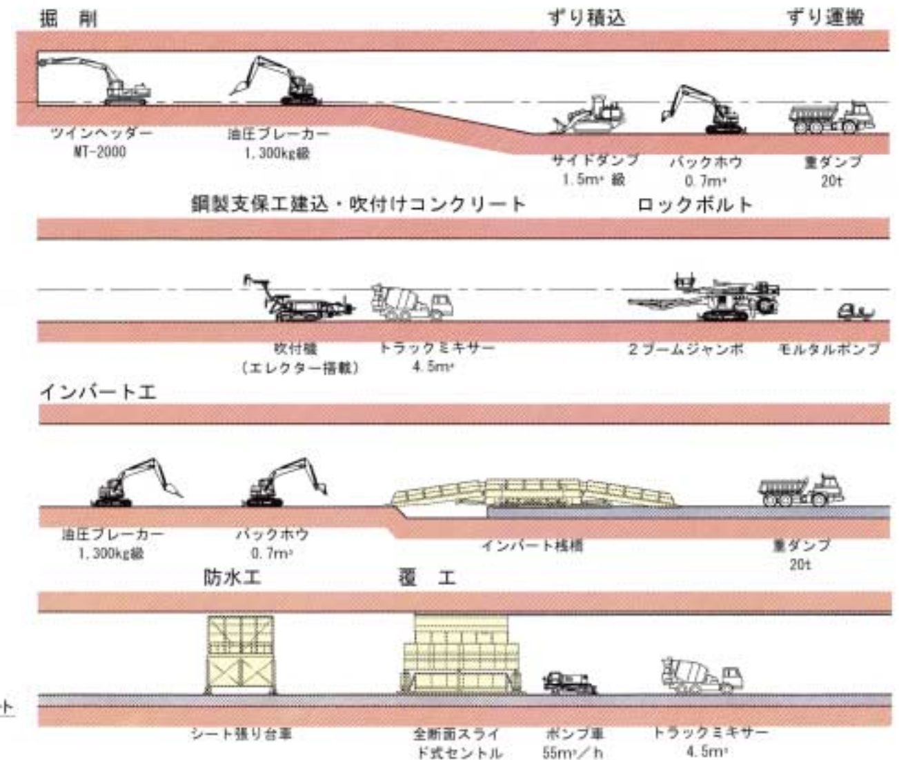
施工順序図
