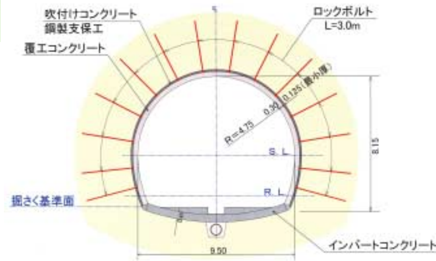
標準支保パターン図
